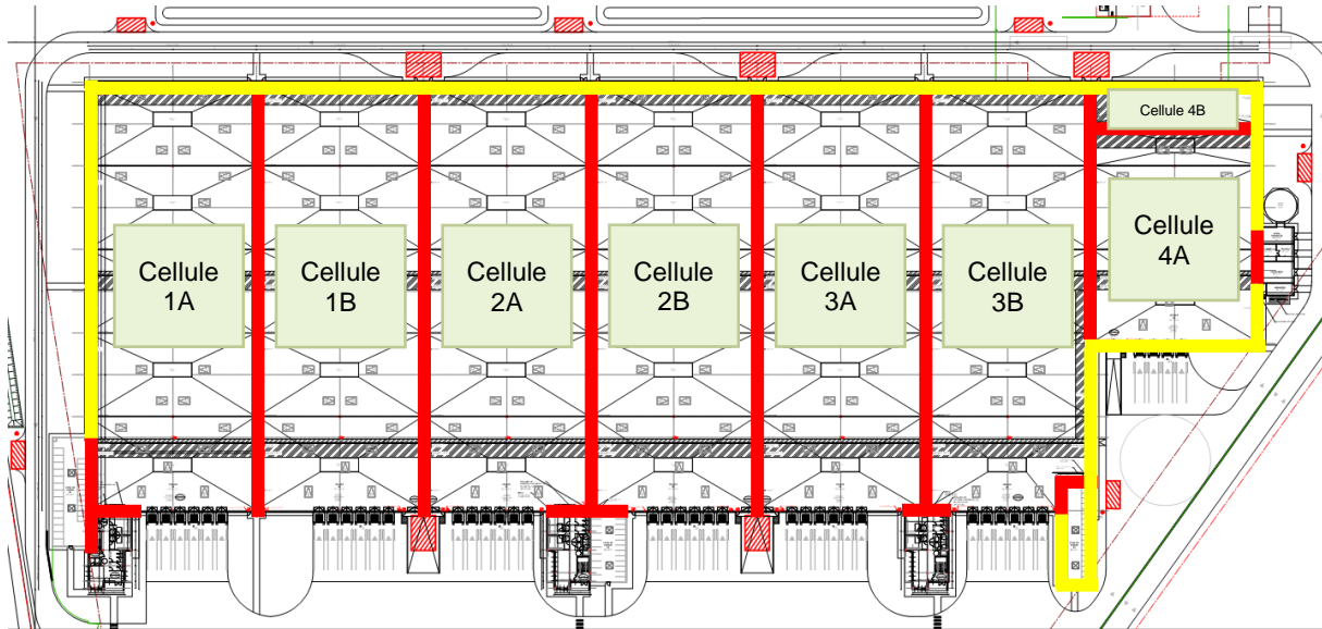
Plan des murs coupe-feu
